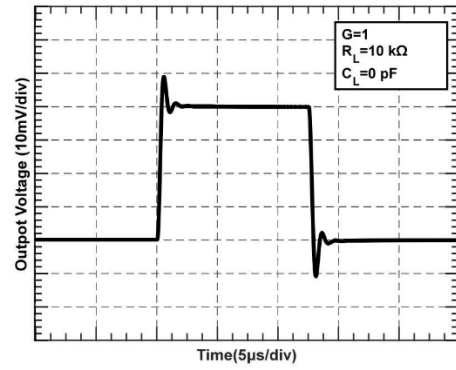
图 4 小信号阶跃响应
